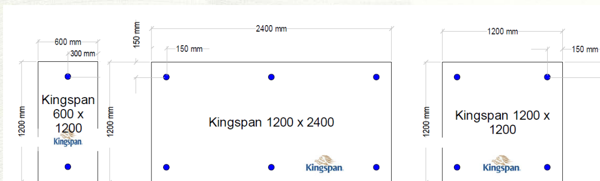
Figuur 3: Bevestigingspatronen Therma™-systeem niPIR-N
